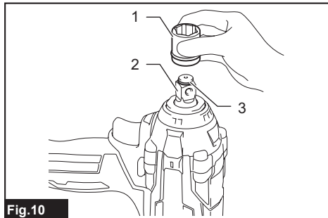
► 1. Douille à choc 2. Tige d'entraînement carrée 3. Ressort annulaire
